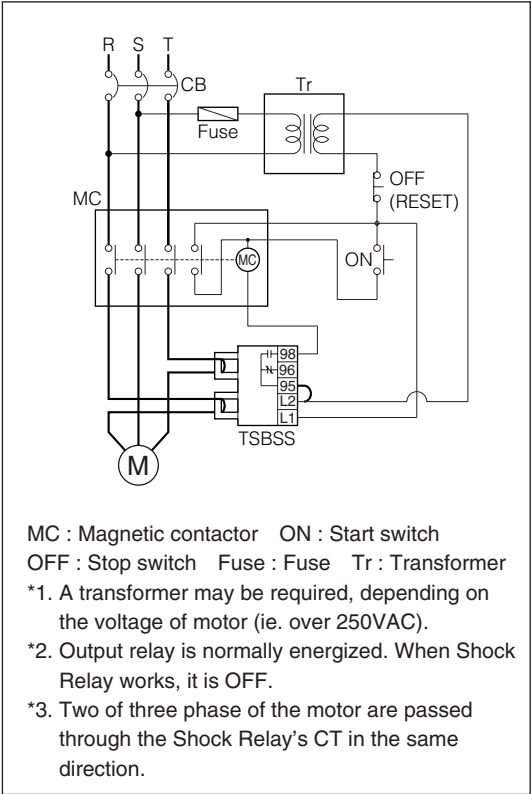
Wiring
